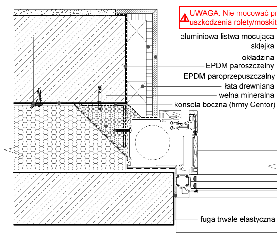
1 detal stojaka ościeżnicy
